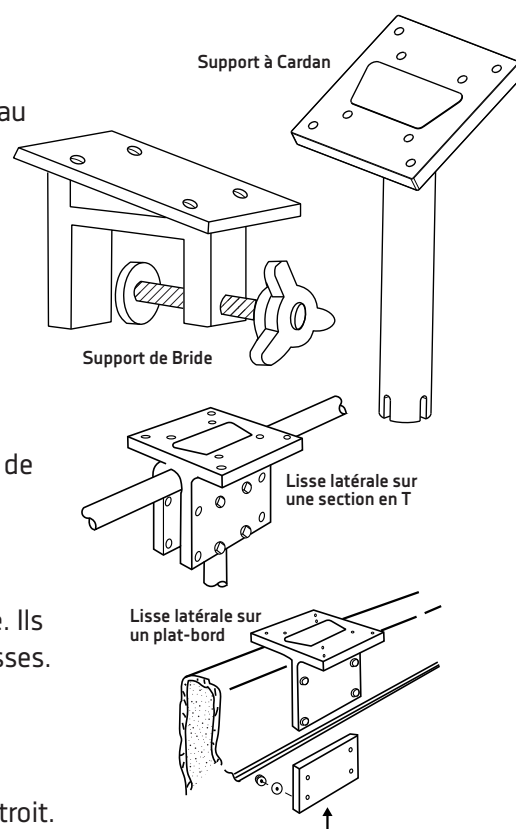
Positions typiques de montage
